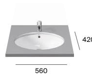
Berna A32787100J 560 x 420
