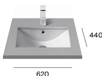
Diverta A32711500J 620 x 440 A32711400J 500 x 380
